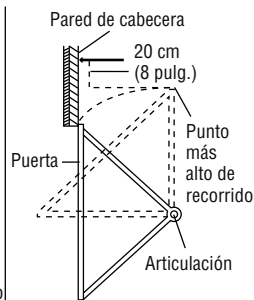
Puerta de una sola pieza sin riel guía: accesorios de articulación
