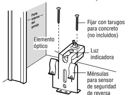
Figura 4 MONTAJE EN PISO (LADO DERECHO)
