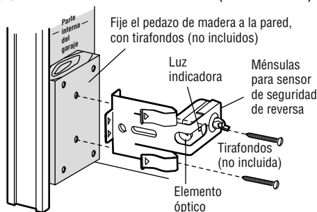
Figura 3 MONTAJE PARED (LADO DERECHO)
