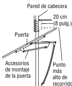
Puerta de una sola pieza sin riel guía: accesorios de montaje
