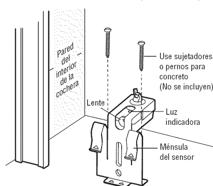
Figura 4 INSTALACIÓN EN EL PISO (LADO DERECHO)
