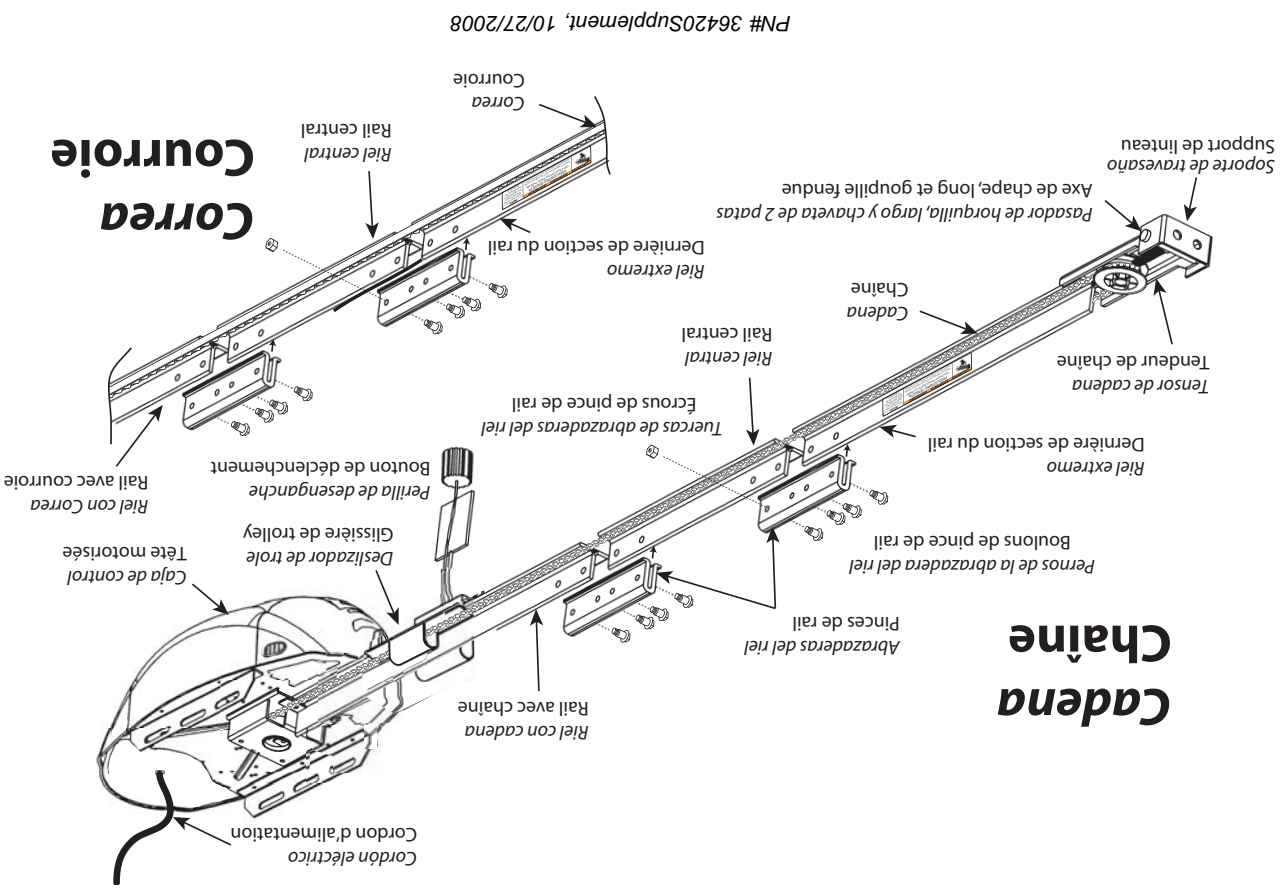
VISTA DEL MONTAJE DE HERRAJES DE RIEL DE 3 PIEZAS VUE DE LA QUINCAILLERIE DU RAIL A 3 PIECES ASSEMBLÉE
