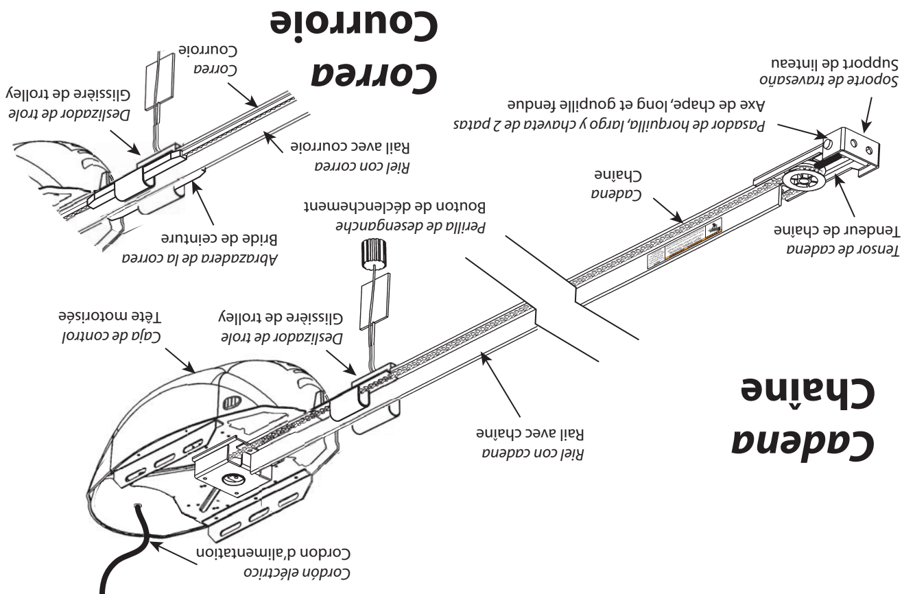
VISTA DEL MONTAJE DE HERRAJES DEL RIEL DE 1 PIEZA VUE DE LA QUINCAILLERIE DU RAIL A 1 PIECE ASSEMBLÉE
