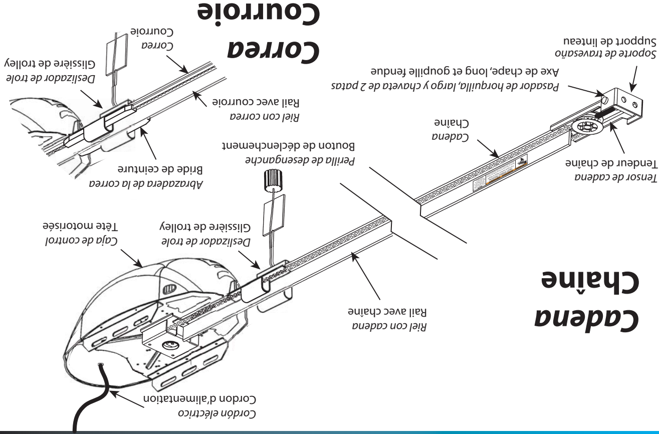
VISTA DEL MONTAJE DE HERRAJES DEL RIEL DE 1 PIEZA VUE DE LA QUINCAILLERIE DU RAIL A 1 PIÈCE ASSEMBLÉE
