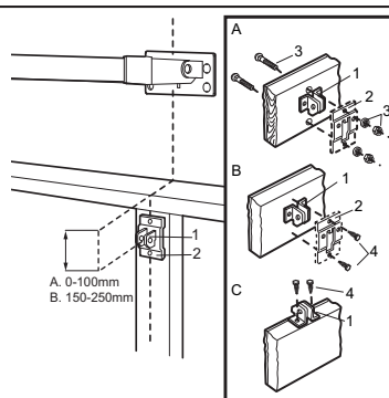
C. Portão de uma folha - opcional Fixe por meio de parafusos para madeira (4).
