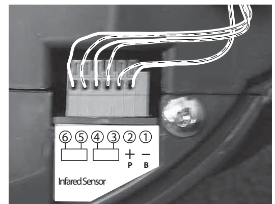
FIG. 4-8 Insert wires
