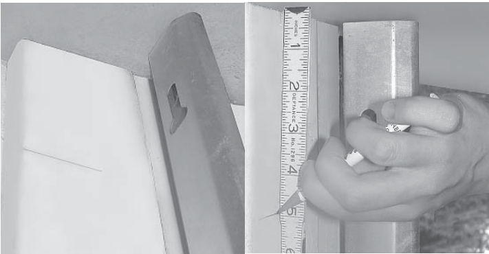
FIG. 4-1 Marque el marco de la puerta
