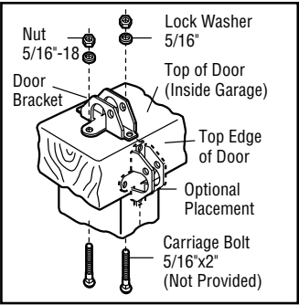
WOOD DOOR
