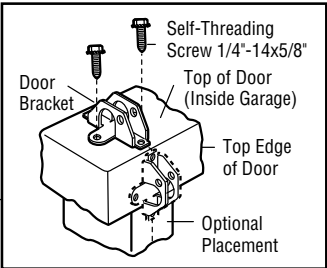
METAL DOOR
